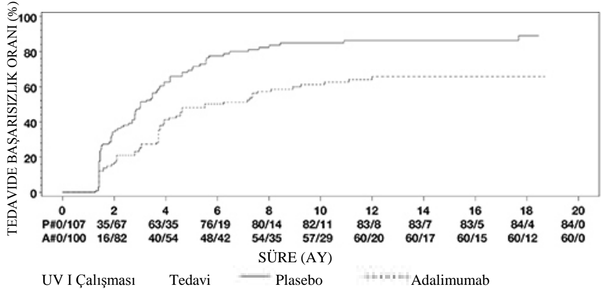
Şekil 1: 6. hafta veya sonrasında ( UV I Çalışması ) ya da 2. hafta veya sonrasında (UV II Çalışması) Tedavide Başarısızlık Ortaya Çıkana Kadar Geçen Süreyi Özetleyen Kaplan-Meier Eğrileri
